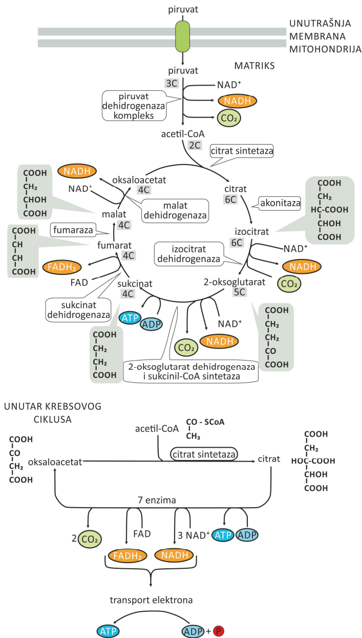
Slika 54. Krebsov ciklus
