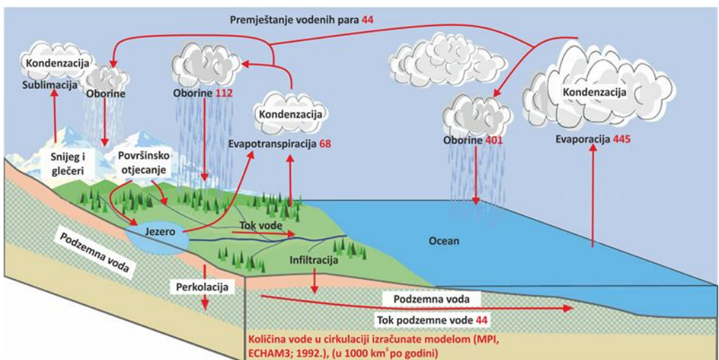
Slika 5. Hidrološki ciklus
